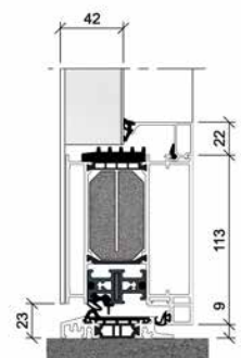
KÖSTER ADVANCE 108 optionale Ausführung mit schrägem Blendrahmen
