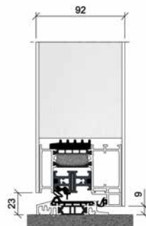
KÖSTER ADVANCE 88 mit einem 75 mm Blendrahmen
